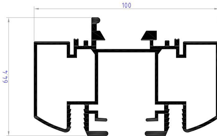
FUT 28 weight 2.138 kg/ml
