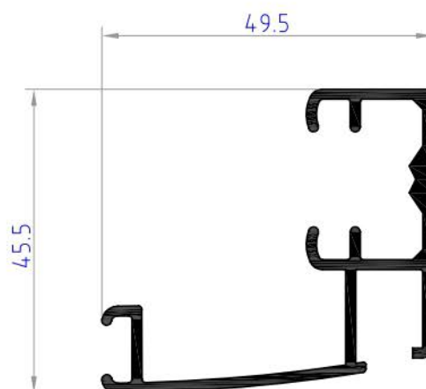
FUT 23 weight 0.641 kg/ml
