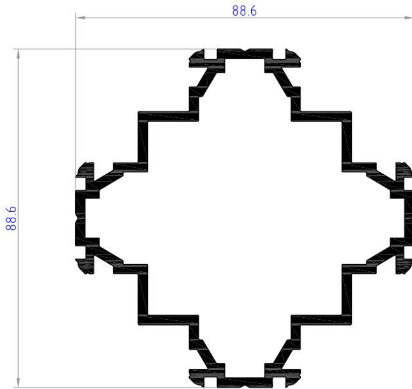
FUT 27 weight 2.522 kg/ml
