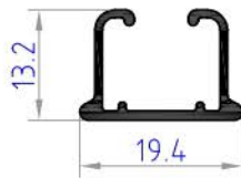
NMK14 weight 0.150 kg/m
